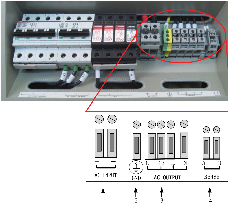
图 3 SG10K3 外部接口示意图
