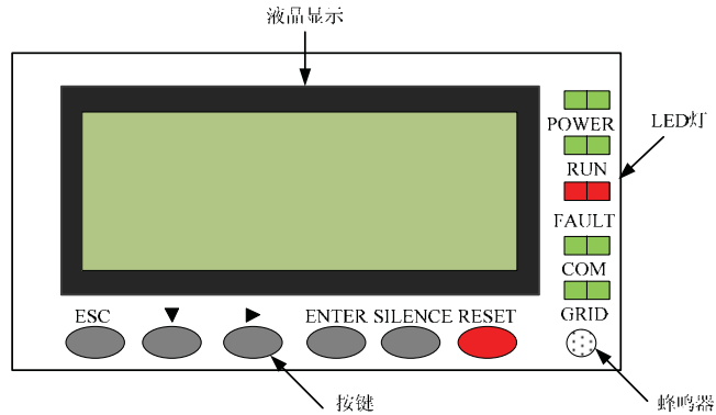
图7 液晶控制面板
