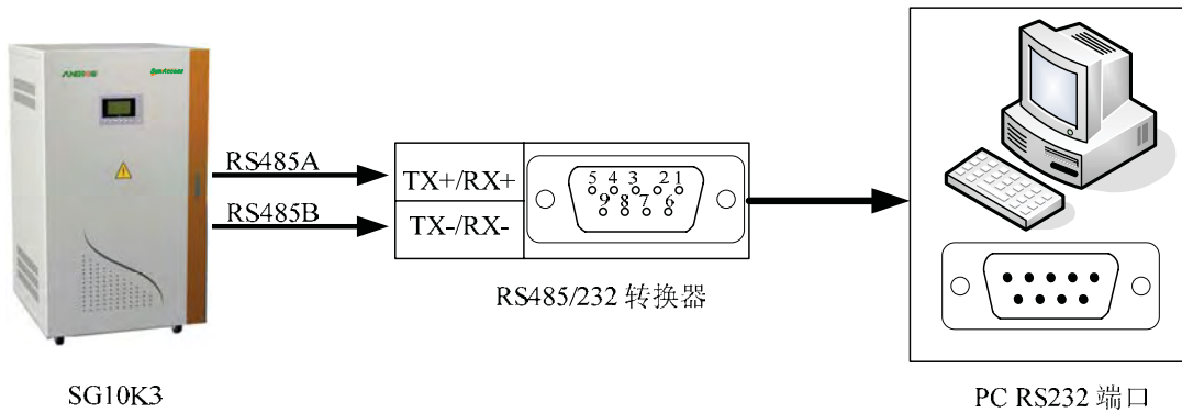
图 11 通讯连接
