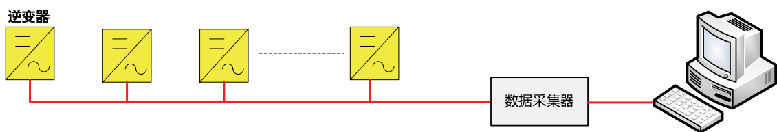
图 6 数据采集器和 PC 机通过 RS485 进行监控
