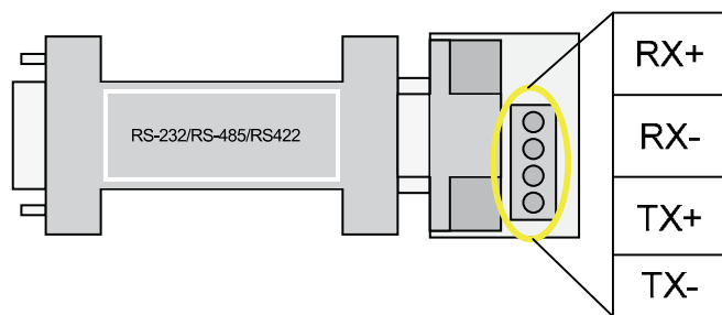
图 12 RS485/RS232 转换器
