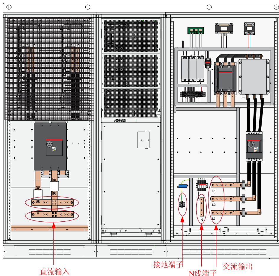
图4-6 接线端子示意图
