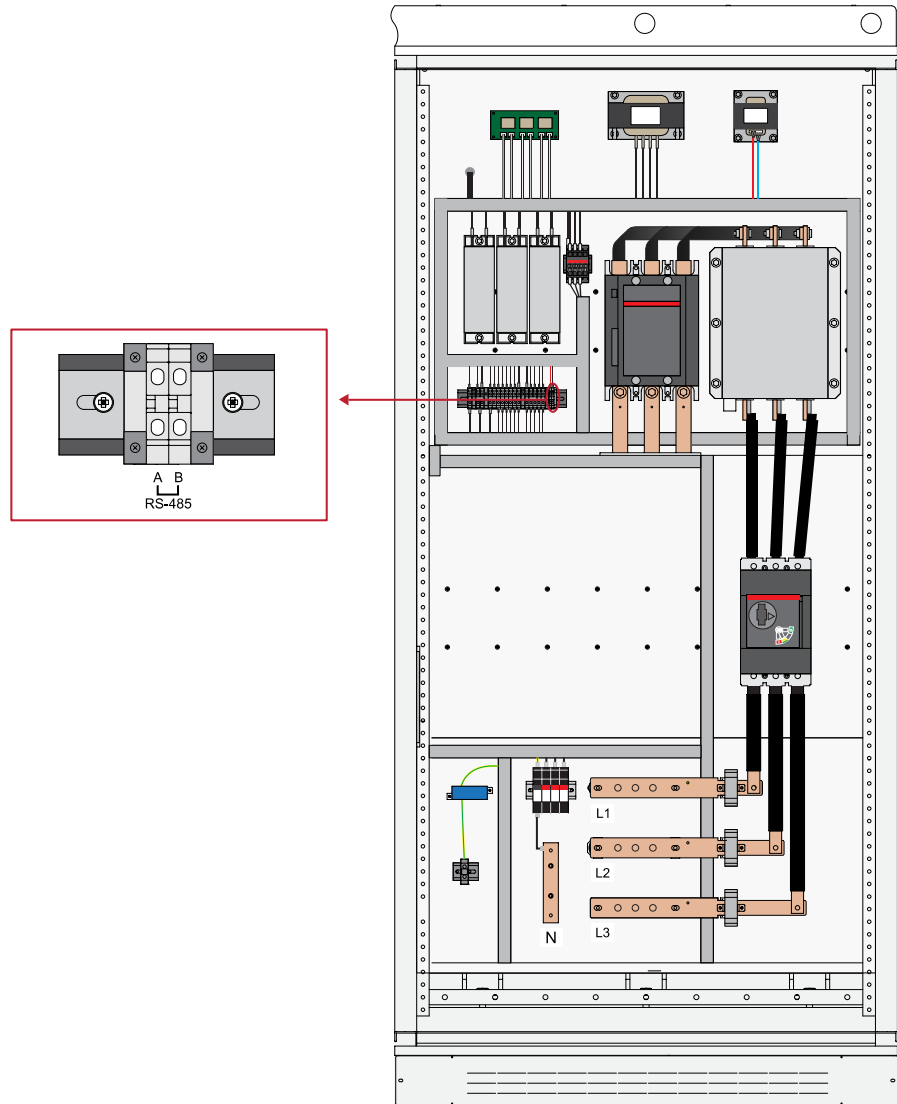
图8-7 通讯系统接线图
