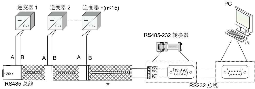
图8-9 PC 机通过 RS485 进行监控
