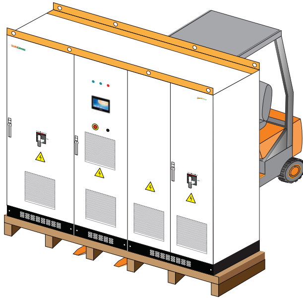
图7-2 叉车运输
