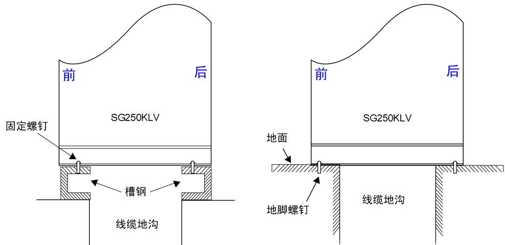
图7-6 逆变器固定方法
