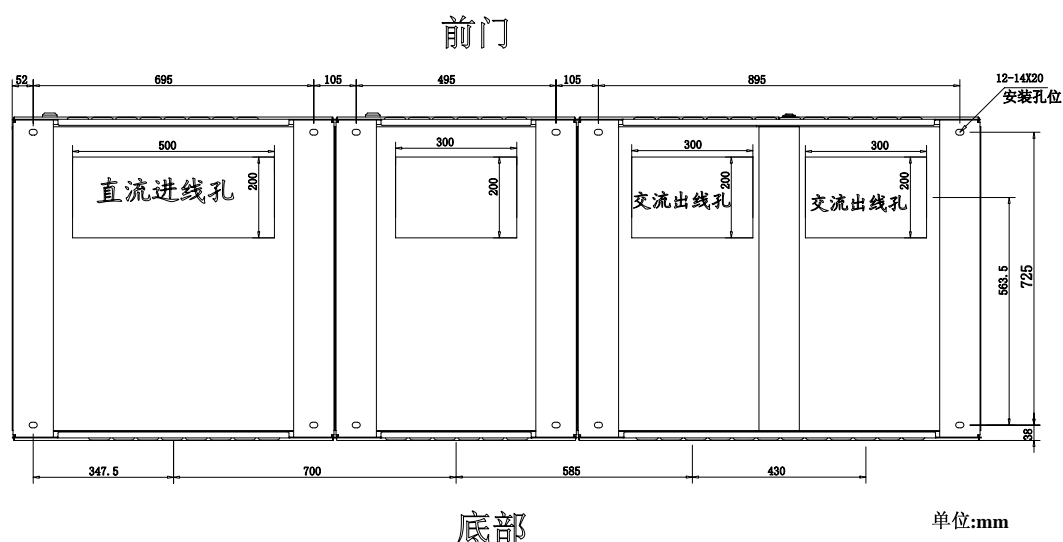
图4-2 SG250KLV 底部视图
