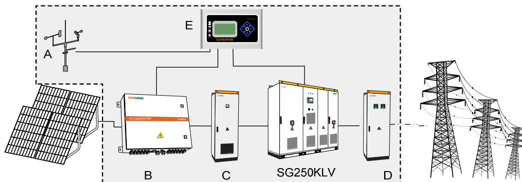
图5-1 光伏并网发电系统可选配置
