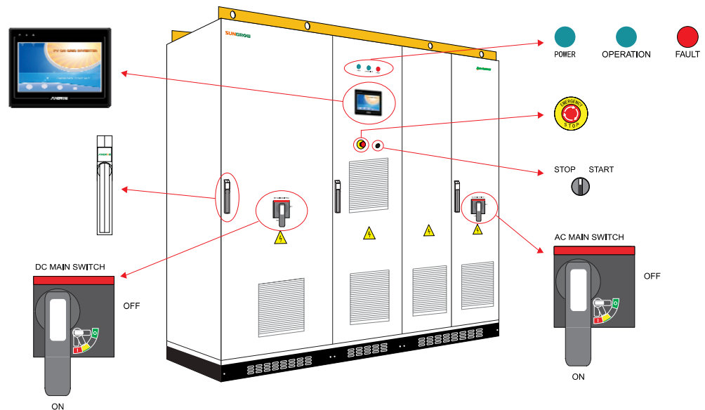
图4-4 SG250KLV 外观图
