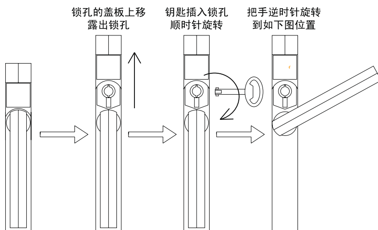
图8-3 开启前门
