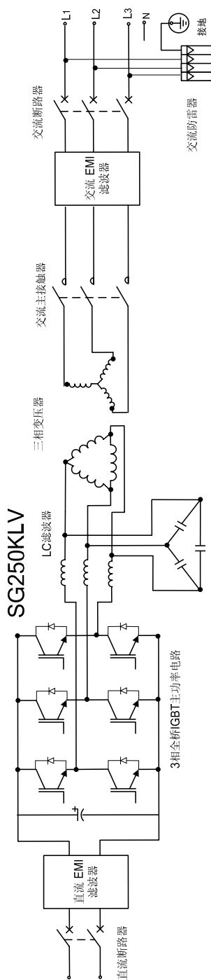
图4-5 SG250KLV 主电路
