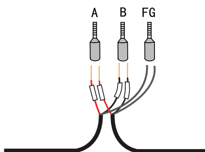
图8-11 端子压线示意
