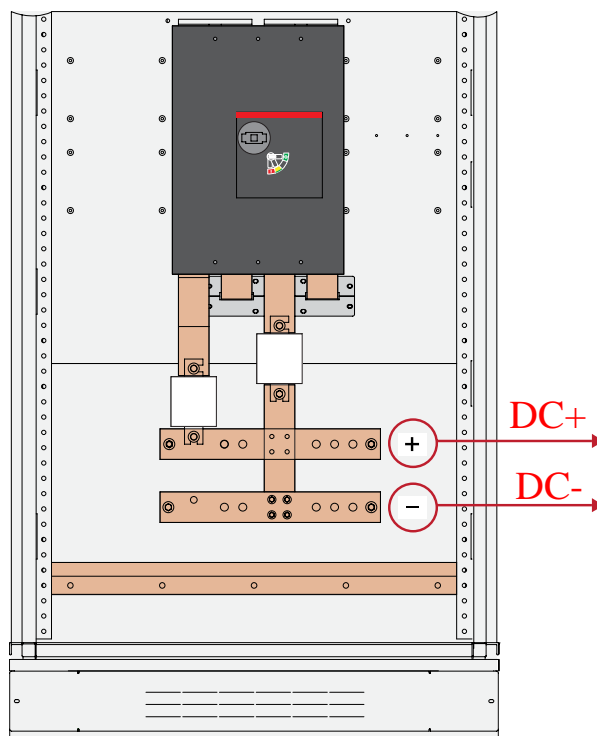
图8-4 直流侧接线端子
