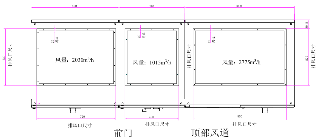
图4-3 顶部出风口
