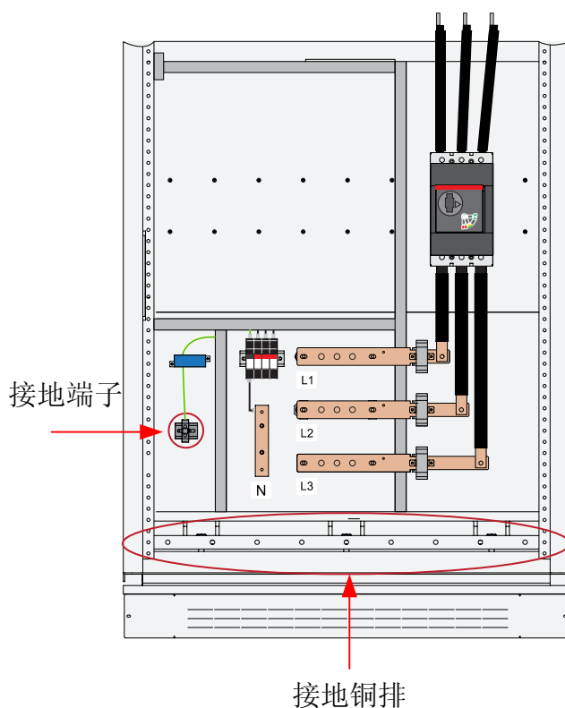
图8-6 接地铜排示意图
