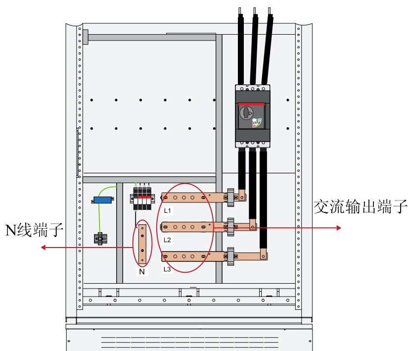
图8-5 交流侧接线端子
