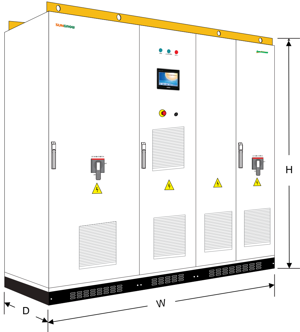
图4-1 整机外观尺寸图
