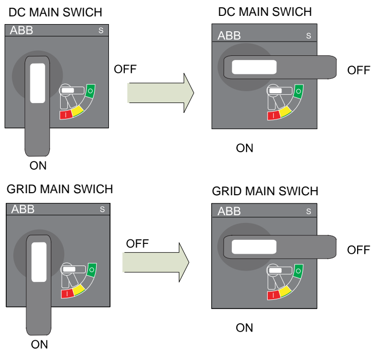
图8-2 关闭断路器
