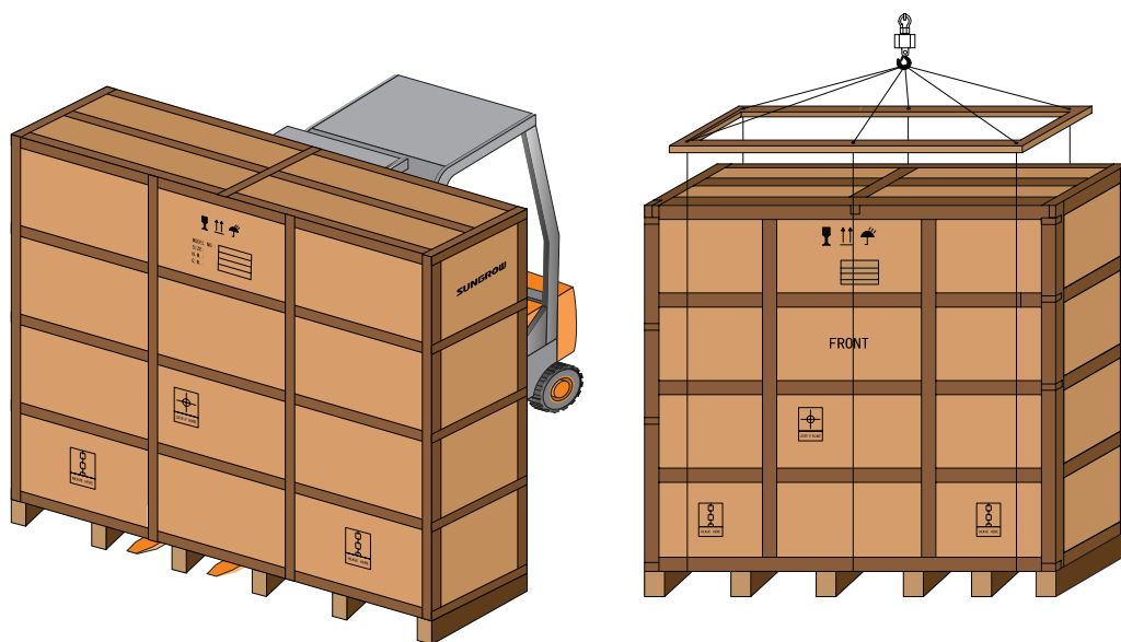
图7-1 带包装逆变器运输
