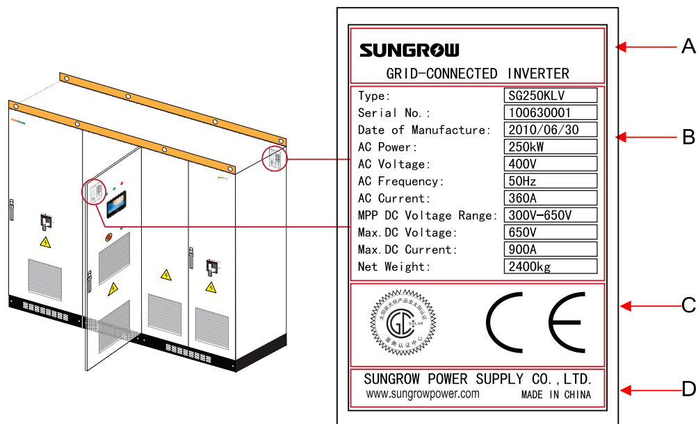
图3-1 SG250KLV 铭牌及位置示意（图片仅供参考，请以实物为准）
