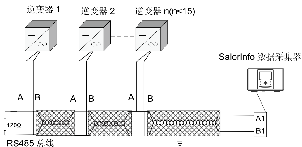
图8-8 数据采集器通过 RS485 进行监控
