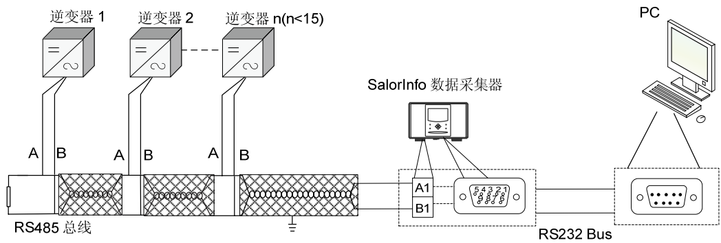
图8-10 数据采集器和 PC 机通过 RS485 进行监控
